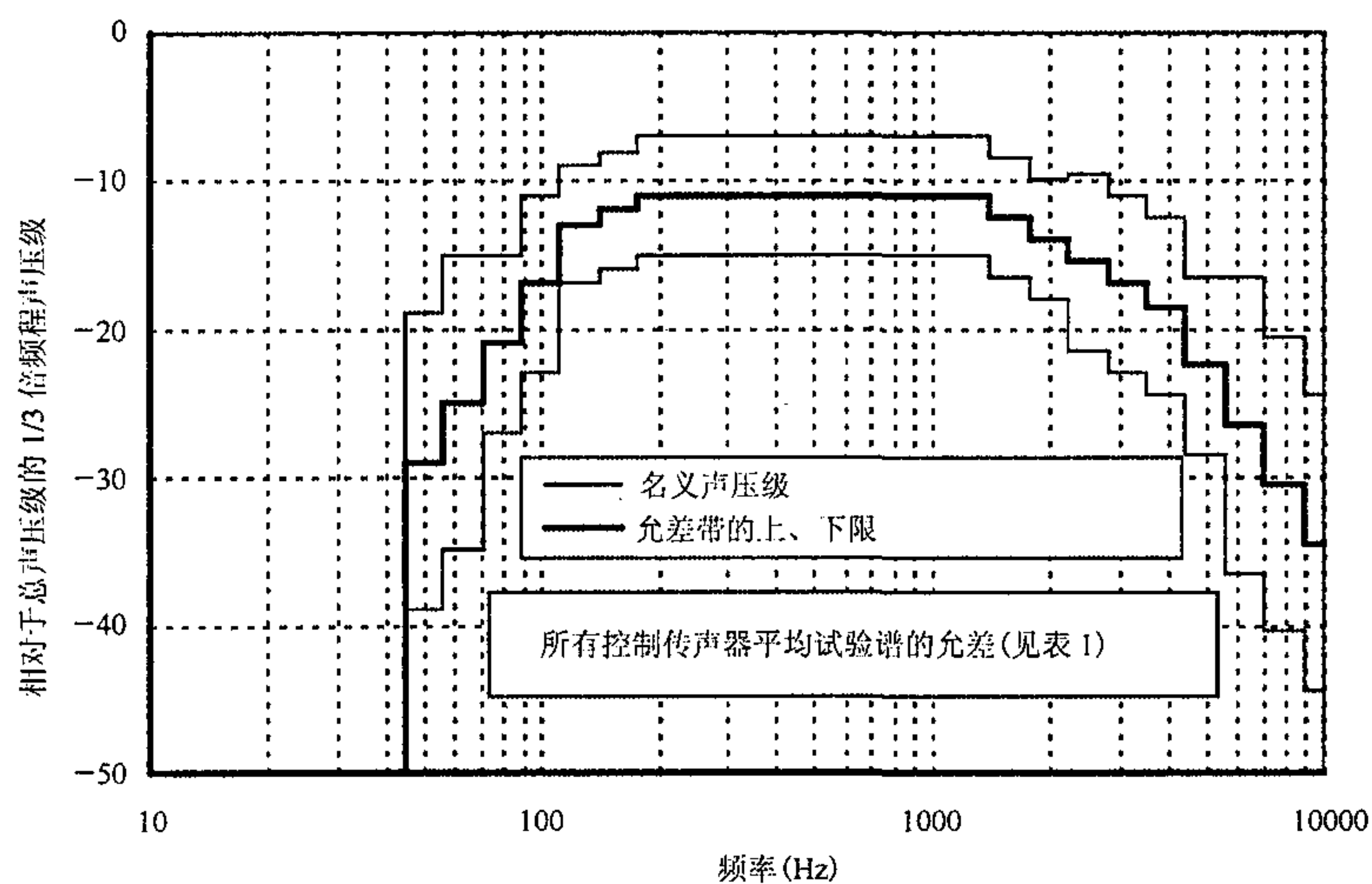
图 B.1 施加的试验谱
